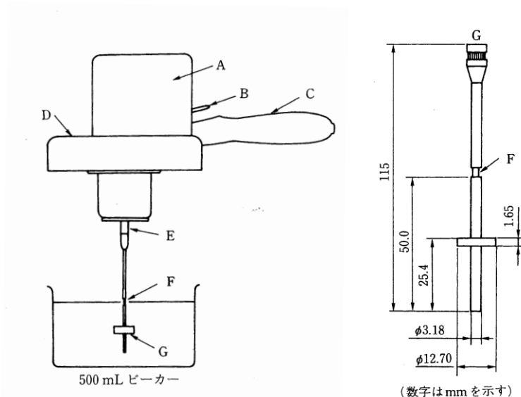
ブルックフィールド型粘度計
